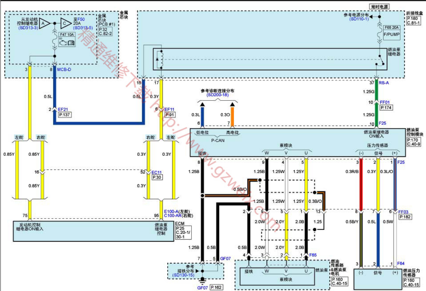
发动机控制系统(G6DG/G6DH/G6DJ:LAMBDA II 3.0L/3.3L/3.8L GDI)(4)
